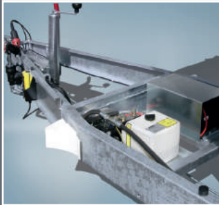
Handpumpe + Fernbedienung
