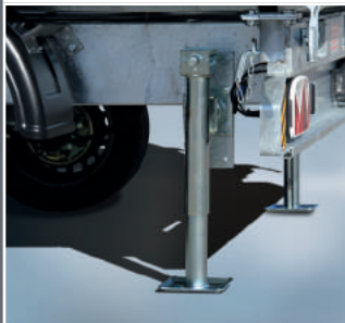
Drehkurbelstütze
